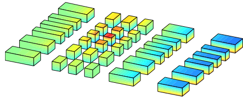
\sigma_{xx}
