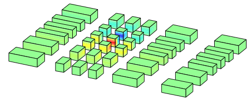
\sigma_{yz}
